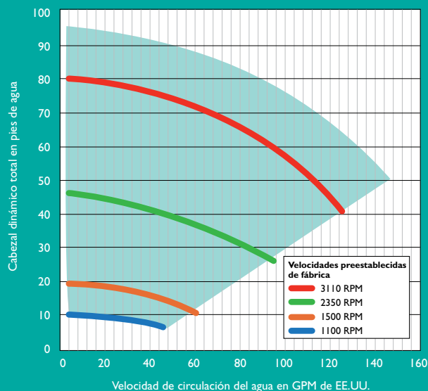
Curvas de rendimiento de la bomba
