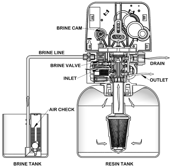
15. Brine/Slow Rinse Position
